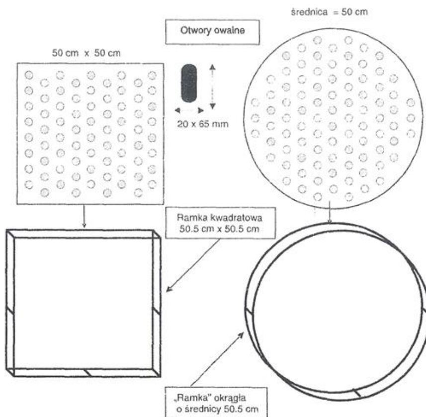
Rys. 1. Konstrukcja sit kwadratowych lub okrągłych.
